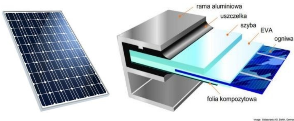
Rysunek 1. Pojedynczy moduł fotowoltaiczny oraz jego przekrój.
